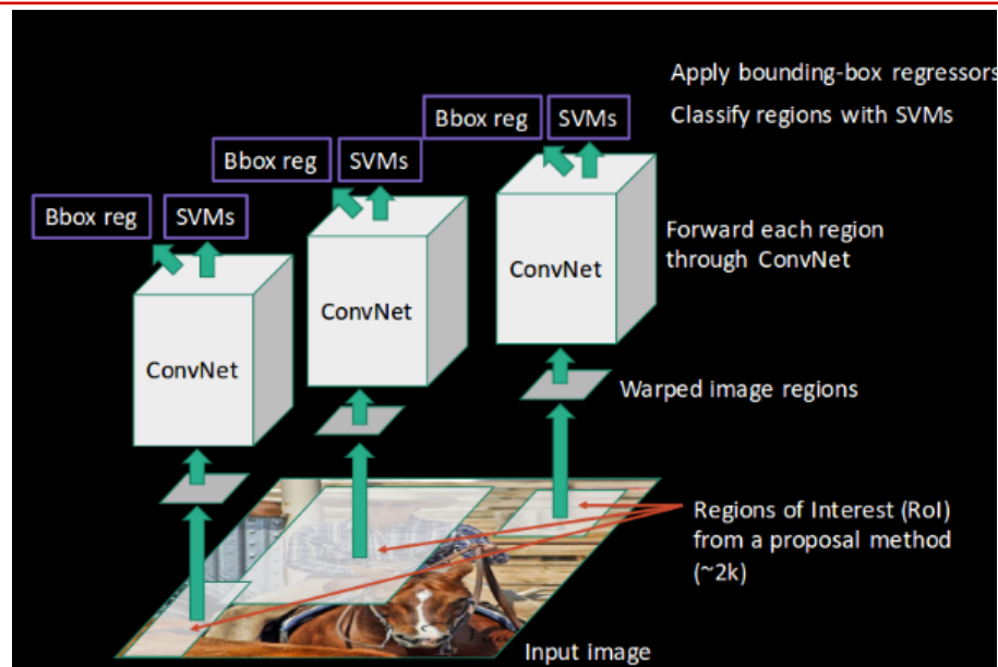
R-CNN
