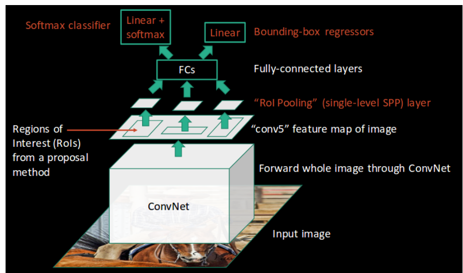
Fast R-CNN
